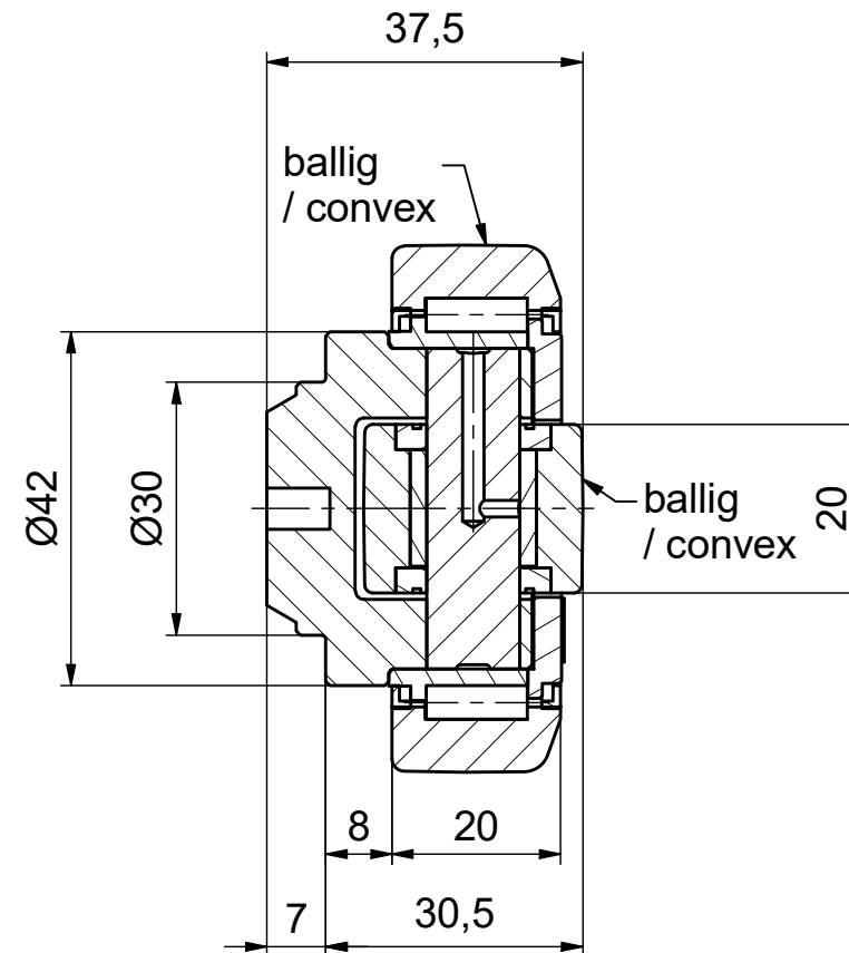
A-A ( 1 : 1 )
