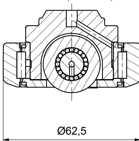
B-B ( 1 : 1 )
