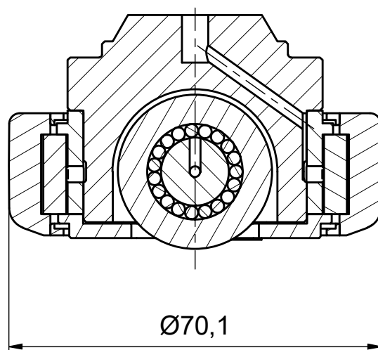
B-B ( 1 : 1 )
