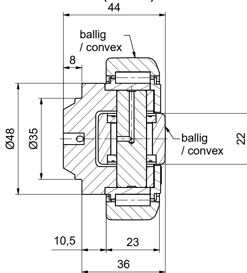
A-A ( 1 : 1 )
