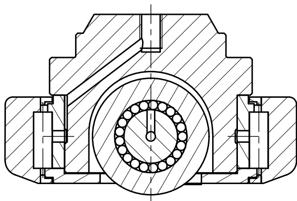
B-B ( 1 : 1 )
