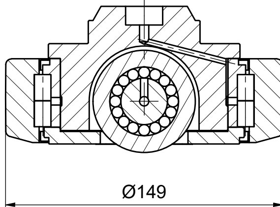
B-B ( 1 : 2 )
