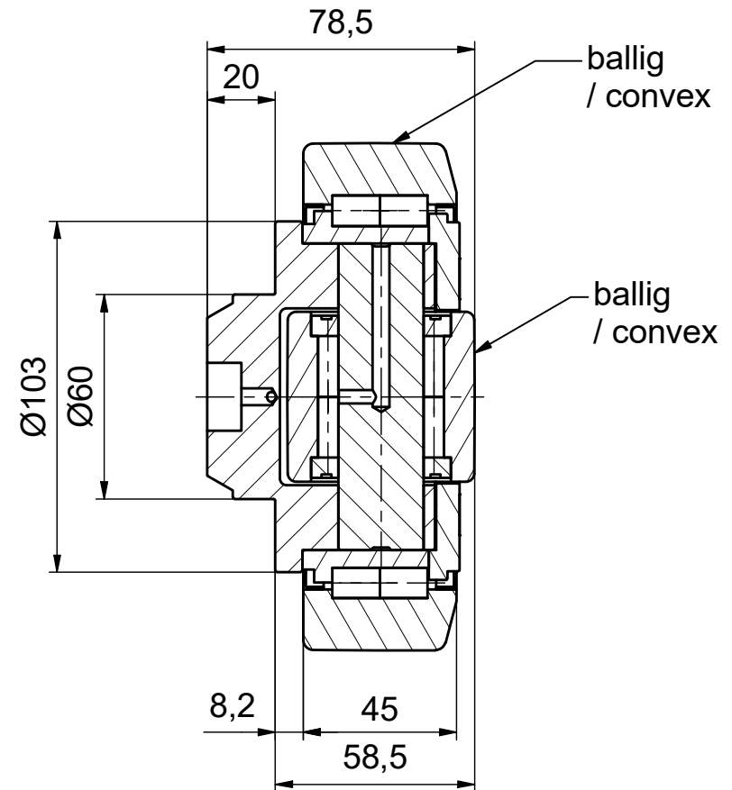
A-A ( 1 : 2 )
