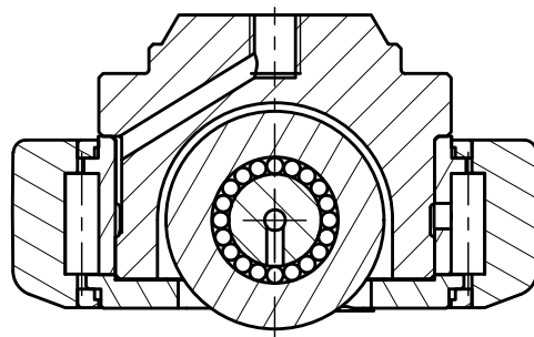
B-B ( 1 : 1 )
