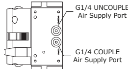
VIEW A-A
