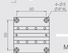
MX(Y)60-A Mounting Dimensions
