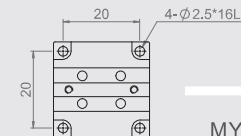
MX(Y)25-A Mounting Dimensions
