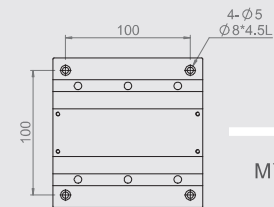
MX(Y)120-A Mounting Dimensions
