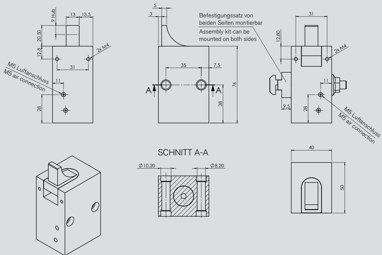
D0-400-09-EW-V
